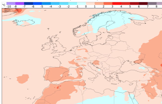
Temperaturentwicklung 03.11. - 10.11. (Woche 4)
