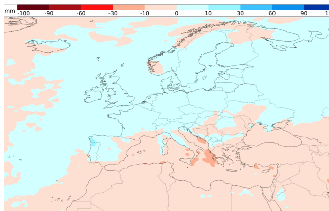
Niederschlagsentwicklung 03.11. - 10.11. (Woche 4)
