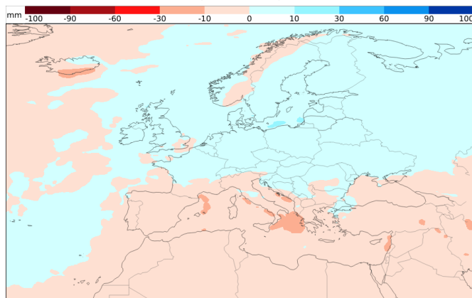
Niederschlagsentwicklung 27.10. - 03.11. (Woche 3)
