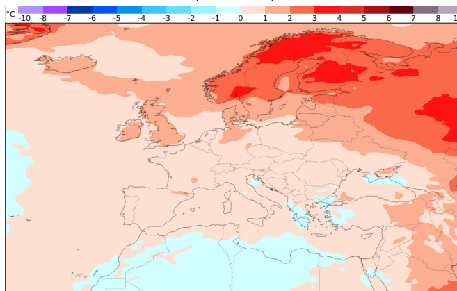
Temperaturentwicklung 15.12. - 22.12. (Woche 4)
