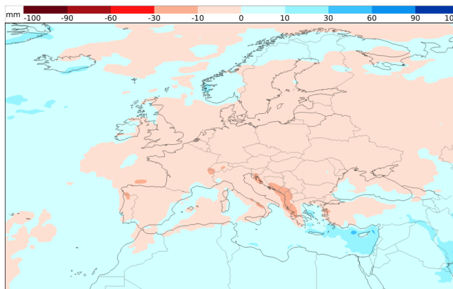
Niederschlagsentwicklung 15.12. - 22.12. (Woche 4)
