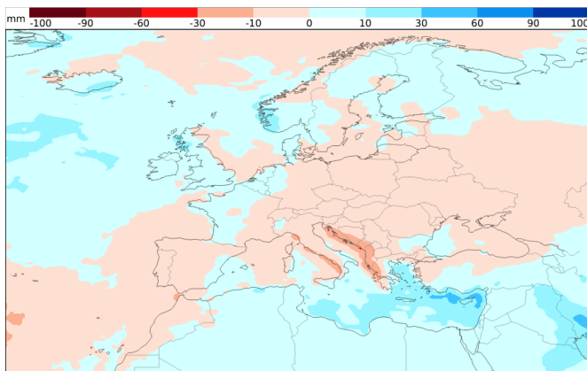
Niederschlagsentwicklung 08.12. - 15.12. (Woche 3)
