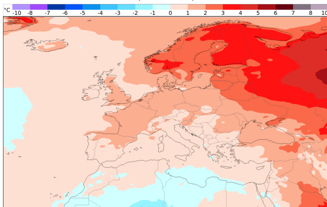
Temperaturentwicklung 08.12. - 15.12. (Woche 3)
