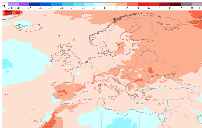
Temperaturentwicklung 15.09. - 22.09. (Woche 3)
