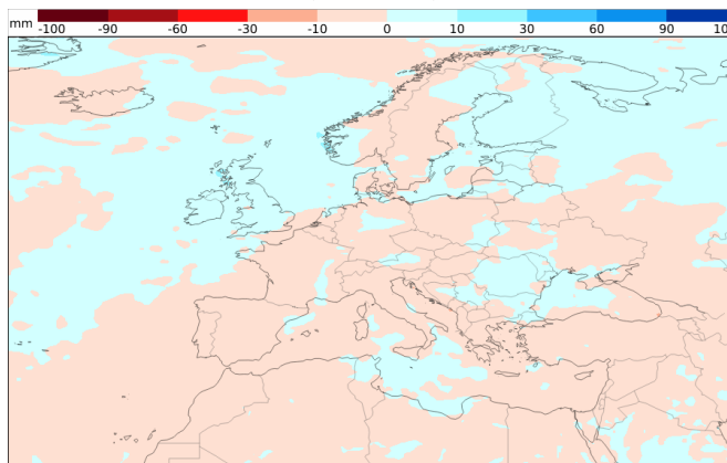
Niederschlagsentwicklung 22.09. - 29.09. (Woche 4)
