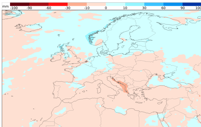
Niederschlagsentwicklung 15.09. - 22.09. (Woche 3)
