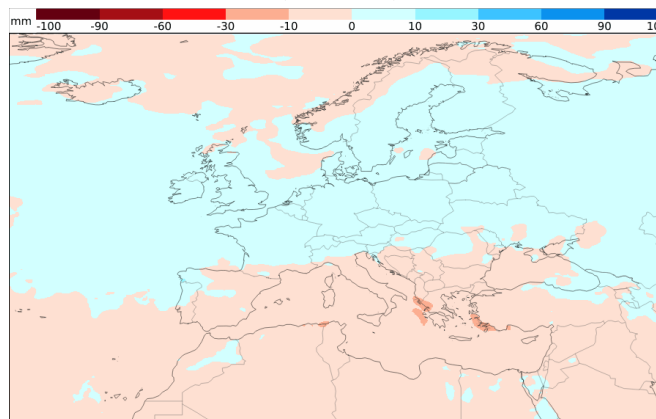
Niederschlagsentwicklung 23.02. - 02.03. (Woche 4)
