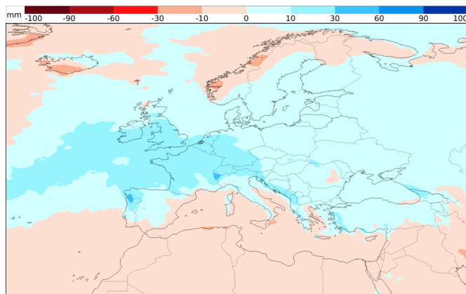
Niederschlagsentwicklung 16.02. - 23.02. (Woche 3)
