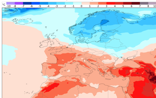
Temperaturentwicklung 16.02. - 23.02. (Woche 3)
