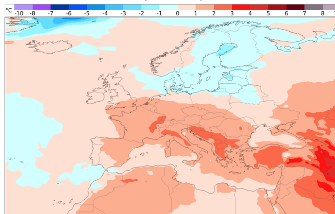
Temperaturentwicklung 23.02. - 02.03. (Woche 4)
