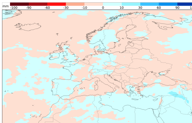
Niederschlagsentwicklung 04.05. - 11.05. (Woche 4)
