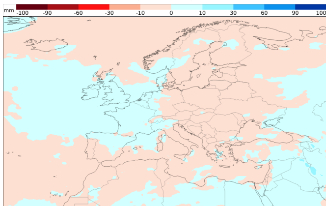
Niederschlagsentwicklung 27.04. - 04.05. (Woche 3)
