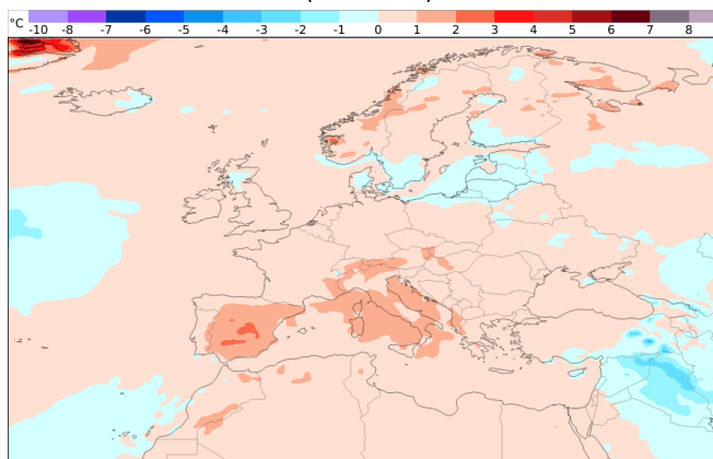
Temperaturentwicklung 04.05. - 11.05. (Woche 4)
