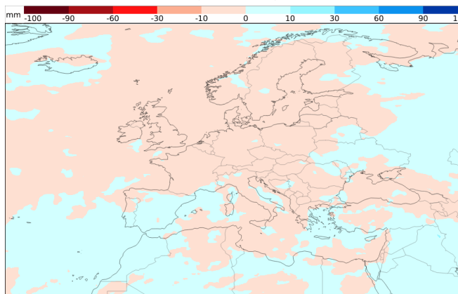
Niederschlagsentwicklung 20.04. - 27.04. (Woche 4)
