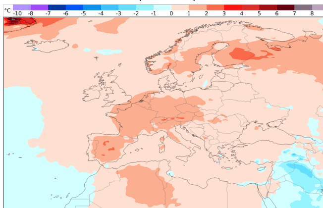
Temperaturentwicklung 20.04. - 27.04. (Woche 4)
