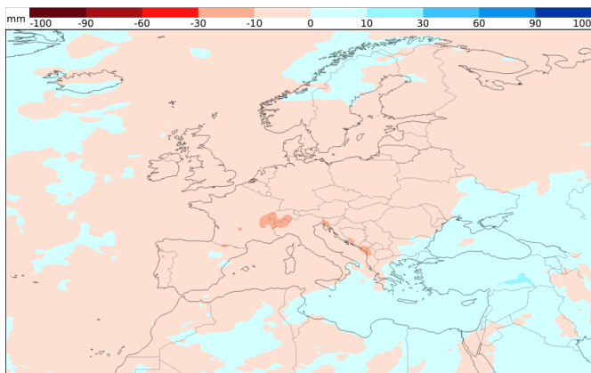
Niederschlagsentwicklung 13.04. - 20.04. (Woche 3)
