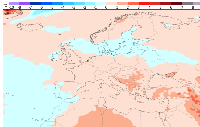
Temperaturentwicklung 09.03. - 16.03. (Woche 4)
