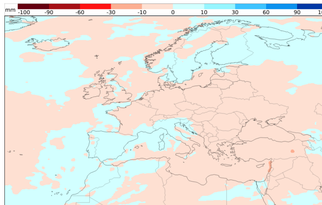
Niederschlagsentwicklung 09.03. - 16.03. (Woche 4)
