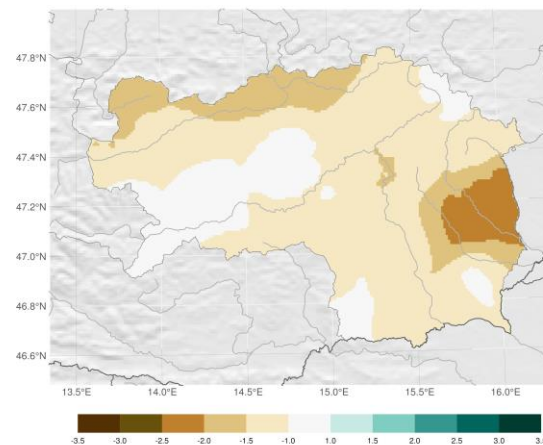
Index der klimatischen Wasserbilanz (Dürreindex) der letzten 30 Tage; Flächenmittel: -1.28
