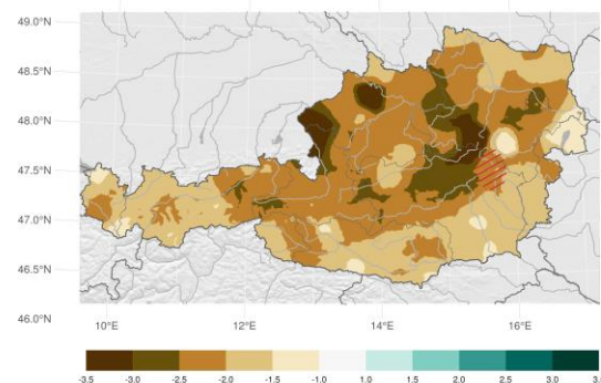
Index der klimatischen Wasserbilanz (Dürreindex) der letzten 30 Tage; Flächenmittel: -1.28
