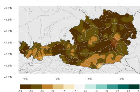
Index der klimatischen Wasserbilanz (Dürreindex) der letzten 365 Tage; Flächenmittel: -2.93
