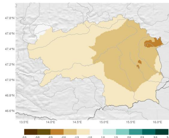
Index der klimatischen Wasserbilanz (Dürreindex) der letzten 30 Tage; Flächenmittel: -1.5
