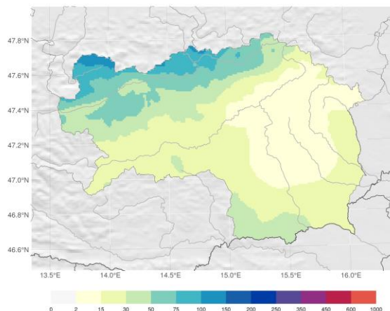
Niederschlagssumme der letzten 30 Tage Flächenmittel: 31.02 mm
