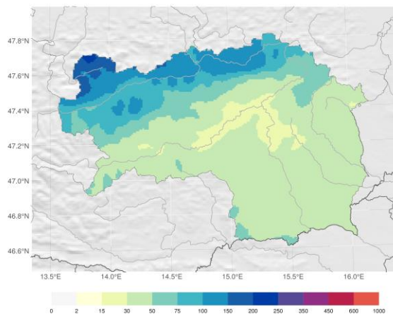
Niederschlagssumme der letzten 30 Tage Flächenmittel: 56.92 mm
