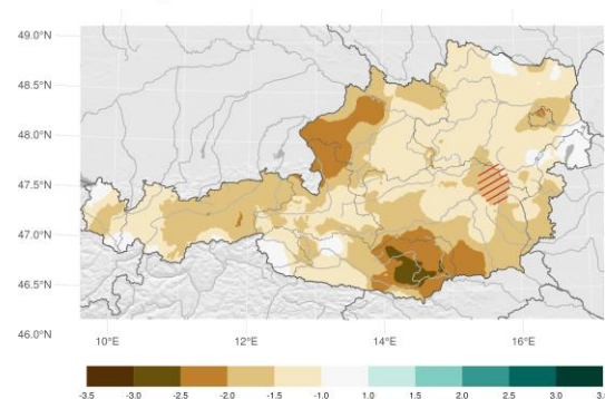
Index der klimatischen Wasserbilanz (Dürreindex) der letzten 365 Tage; Flächenmittel: -1.52
