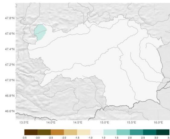
Index der klimatischen Wasserbilanz (Dürreindex) der letzten 30 Tage; Flächenmittel: 0.12
