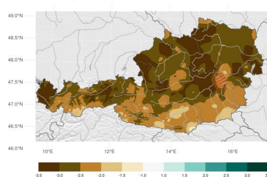
Index der klimatischen Wasserbilanz (Dürreindex) der letzten 365 Tage; Flächenmittel: -2.69
