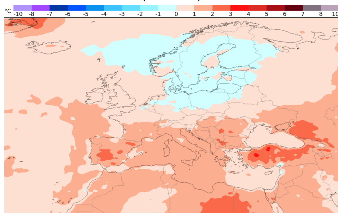
Temperaturentwicklung 14.09. - 21.09. (Woche 3)
