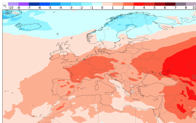
Temperaturentwicklung 24.11. - 01.12. (Woche 3)
