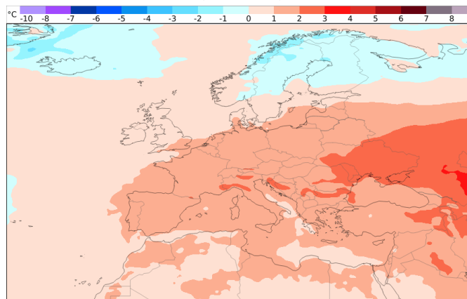
Temperaturentwicklung 01.12. - 08.12. (Woche 4)
