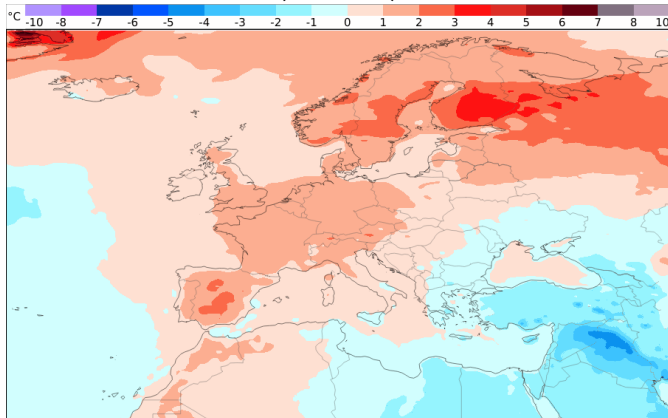
Temperaturentwicklung 13.04. - 20.04. (Woche 3)
