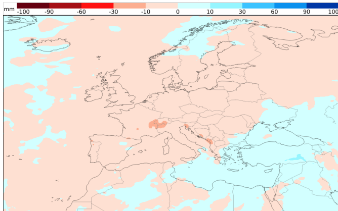
Niederschlagsentwicklung 13.04. - 20.04. (Woche 3)
