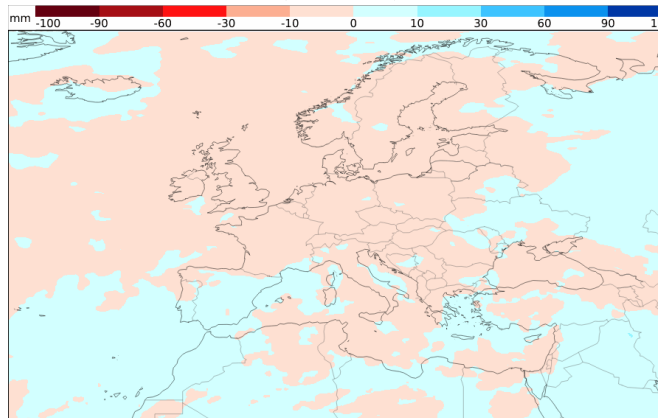
Niederschlagsentwicklung 20.04. - 27.04. (Woche 4)
