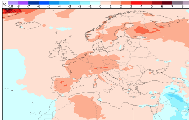
Temperaturentwicklung 20.04. - 27.04. (Woche 4)
