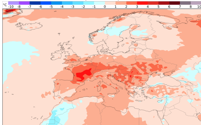
Temperaturentwicklung 06.07. - 13.07. (Woche 3)
