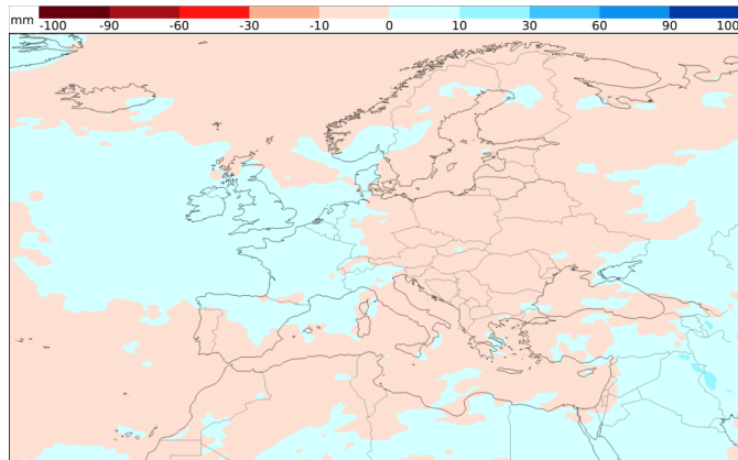
Niederschlagsentwicklung 06.07. - 13.07. (Woche 3)
