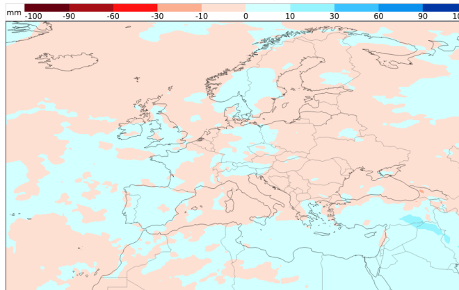
Niederschlagsentwicklung 13.07. - 20.07. (Woche 4)
