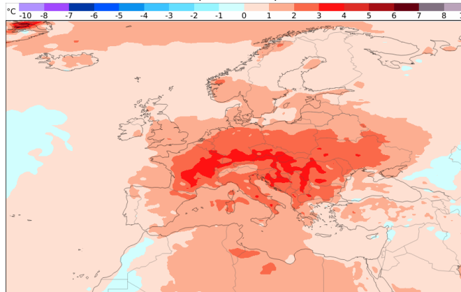
Temperaturentwicklung 13.07. - 20.07. (Woche 4)
