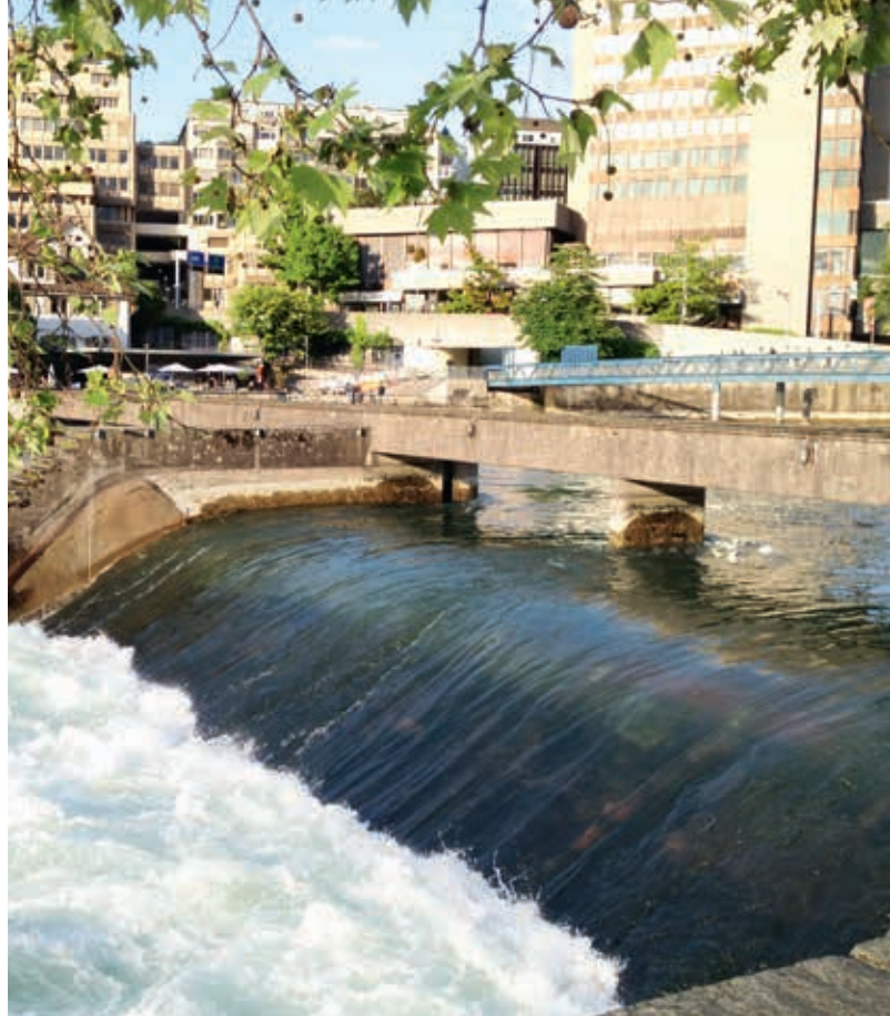
Abb. 8: Lettenwehr – der Seepiegel wird stabilisiert. © AWEL, Kt. Zürich
