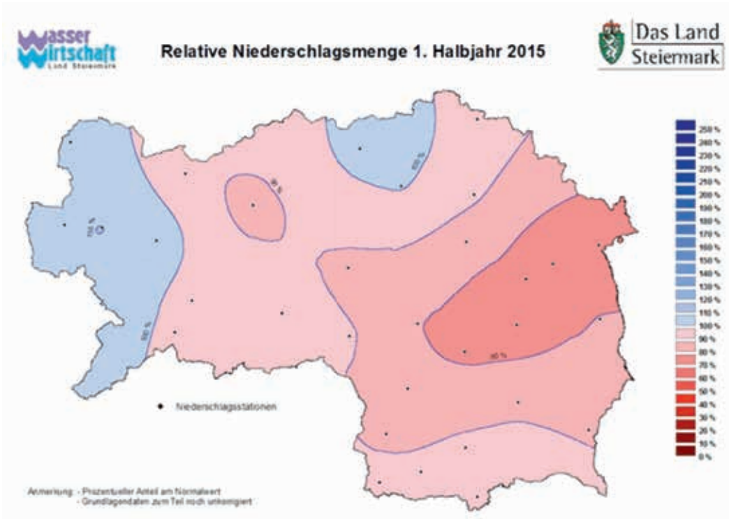
Abb. 2: Relative Niederschlagsmenge in Prozent vom Mittel 1. Halbjahr 2015
